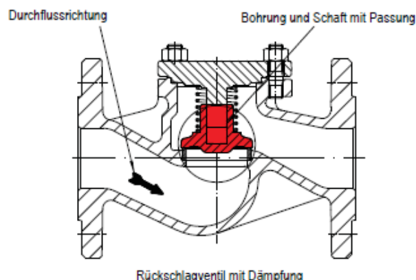
Rückschlagventil mit Dämpfung
